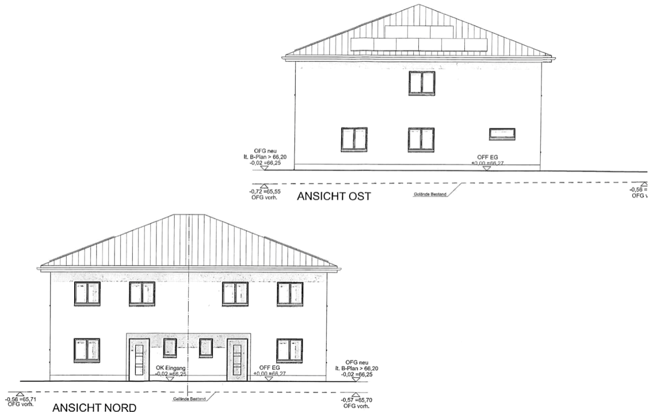
Ansichten Ost & Nord
