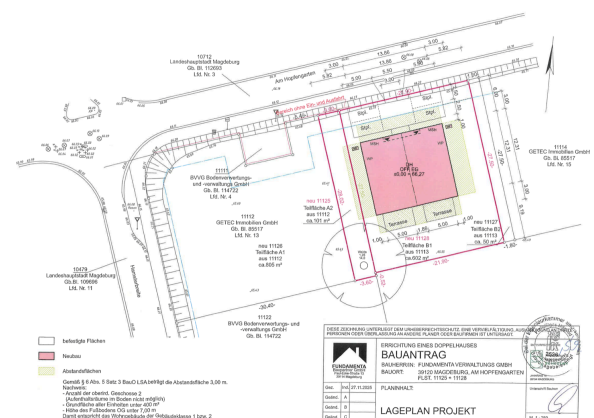
Lageplan / Freiflächen
